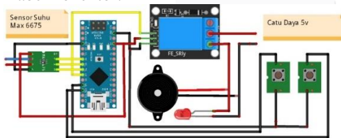
GAMBAR 5. KONFIGURASI RANGKAIAN SENSOR MAX6675 DENGAN ARDUINO NANO
