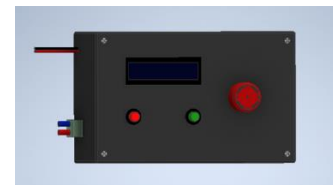
GAMBAR 1. DESAIN 3D ALAT HASIL RANCANGAN
