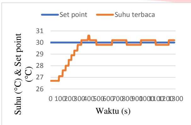
GAMBAR 13 TUNING PID (KP:150, KI:2, KD:2)
