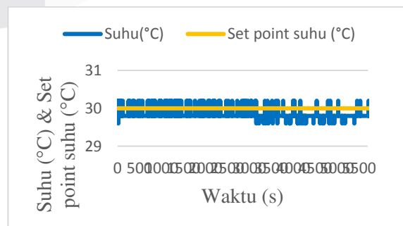
GAMBAR 16 PENGUKURAN SUHU SELAMA 1 HARI
