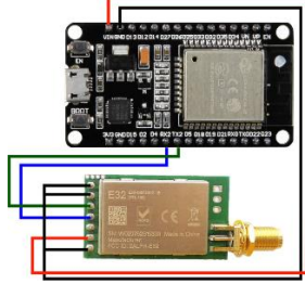
GAMBAR 7 DESAIN RANGKAIAN SISTEM KOMUNIKASI
