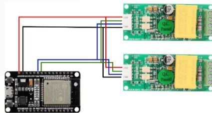
GAMBAR 6 DESAIN RANGKAIAN SISTEM PEMANTAUAN
