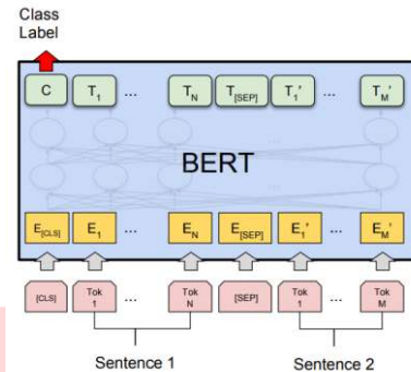
GAMBAR 1 ARSITEKTUR BERT
