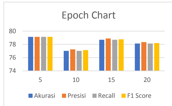
GAMBAR 9 GRAFIK EPOCH
