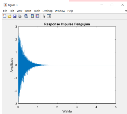
Gambar 4.4 Grafik respon impuls terukur dengan T60_{acuan} = 2 \text{ detik}
