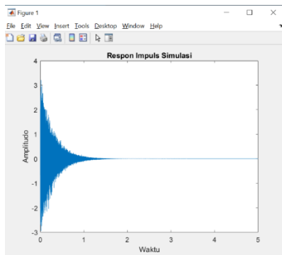
Gambar 4.3 Grafik respon impuls simulasi dengan (T60_{acuan} = 2 \text{ detik})
