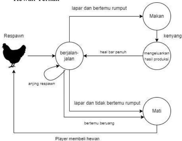
Gambar 4 State Machine Hewan Ternak Perancangan perilaku NPC hewan ternak diatur menggunakan metode FSM, terdapat 4 state pada hewan ternak yaitu wander state, eat seperti gambar diatas. Berikut penjelasannya:
