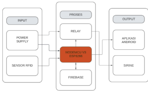
A. DIAGRAM BLOK
