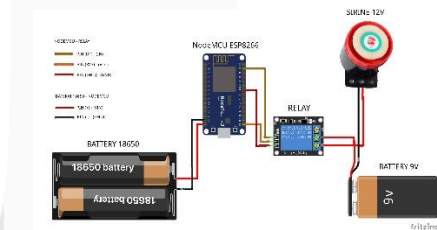
A. PERANCANGAN RANGKAIAN PERANGKAT KERAS
