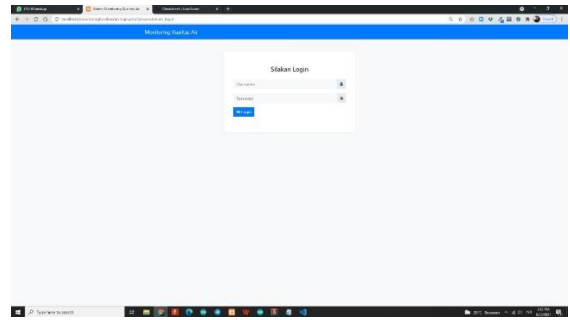
GAMBAR 3.3 HALAMAN LOGIN
