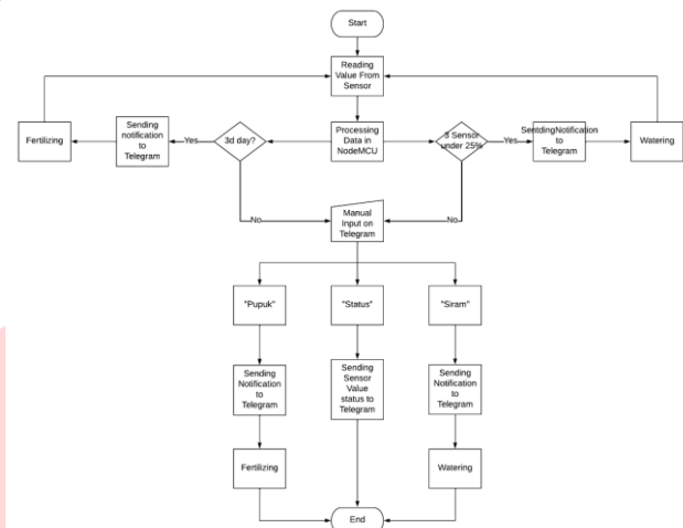
GAMBAR 1. DIAGRAM ALIR SISTEM IOT
