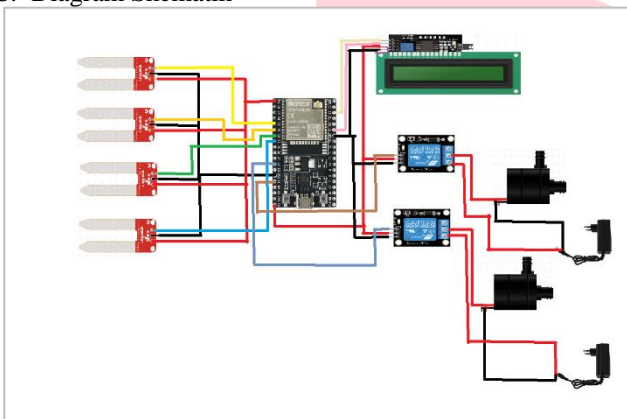
GAMBAR 3. DIAGRAM SKEMATIK
