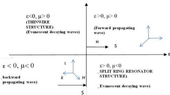
GAMBAR 1. KLASIFIKASI METAMATERIAL.
