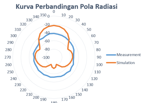
GAMBAR 9 PERBANDINGAN HASIL PENGUKURAN DAN SIMULASI POLA RADIASI
