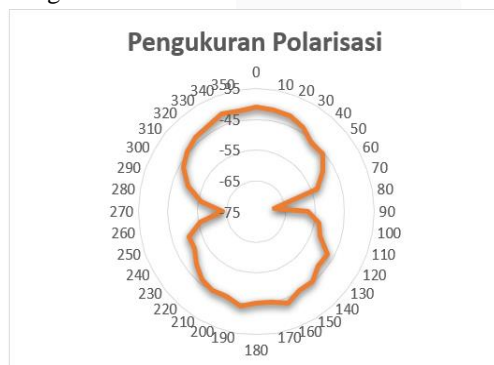
GAMBAR 10 HASIL PENGUKURAN POLARISASI
