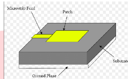
GAMBAR 2 PENCATUAN MICROSTRIP LINE
