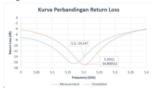
GAMBAR 6 PERBANDINGAN HASIL PENGUKURAN DAN SIMULASI RETURN LOSS
