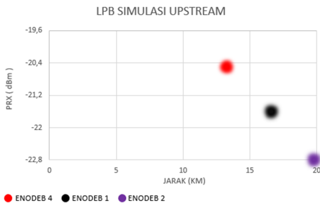
Gambar 5. Hasil Semua LPB Simulasi Upstream
