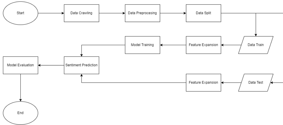
GAMBAR 4 RANCANGAN SISTEM
