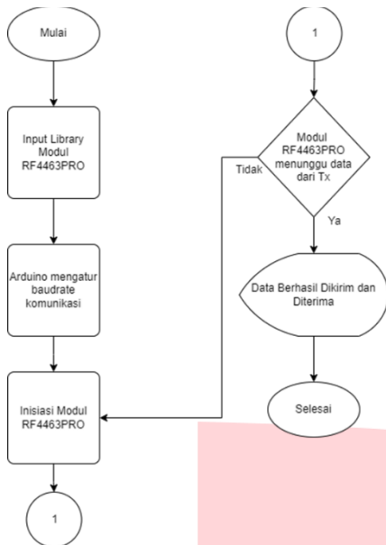
Gambar 7 Algoritma untuk Program Rx
