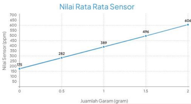
GAMBAR 5 GRAFIK RATA-RATA
