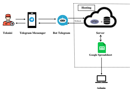
Gambar 2 Blok Diagram Sistem
