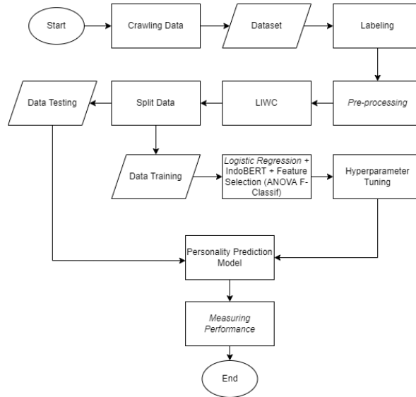
Gambar 1. Sistem Prediksi Kepribadian
