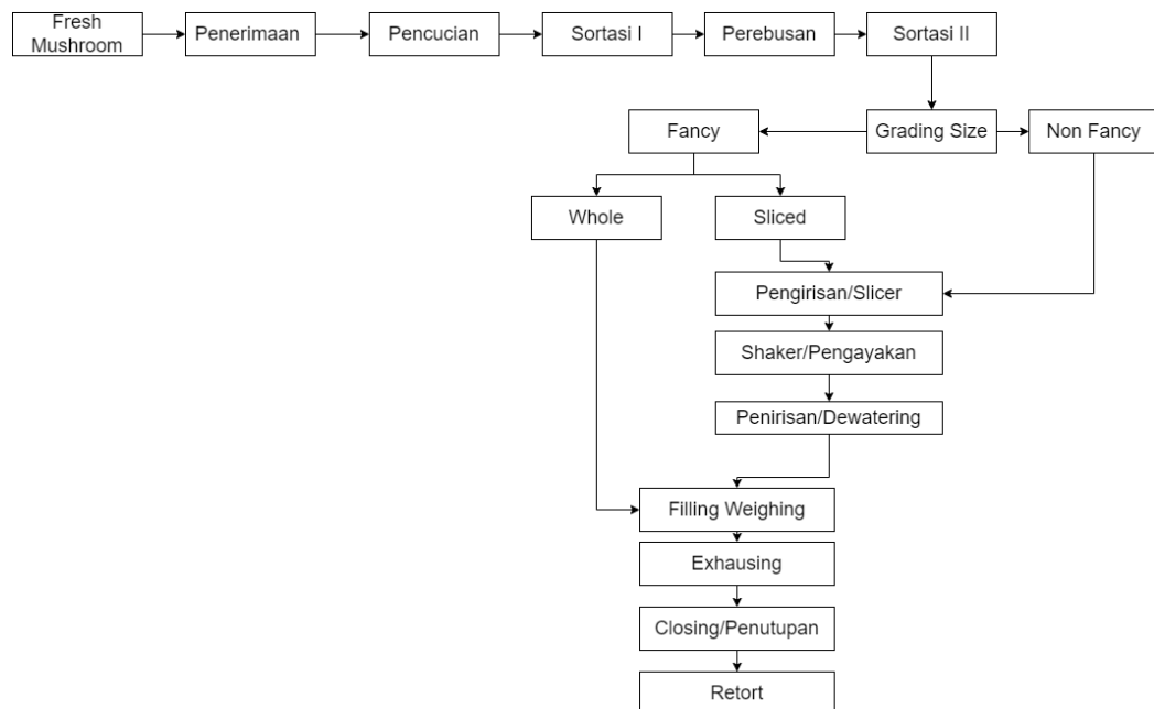
Gambar I.3 Alur Produksi
