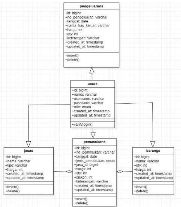
GAMBAR 8 (DESAIN DATABASE)
