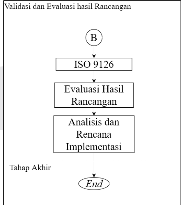
GAMBAR 4 (SISTEMATIKA PERANCANGAN)
