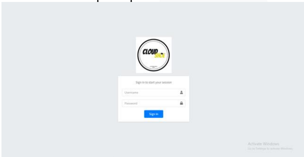
GAMBAR 12 (HALAMAN LOGIN)
