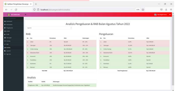
GAMBAR 13 (HALAMAN ANALISIS)
