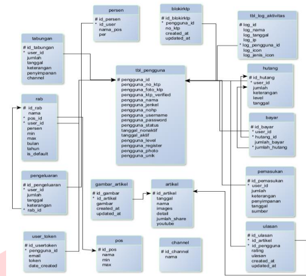
GAMBAR 2 (ERD)
