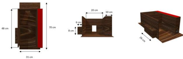
GAMBAR 7 (DIMENSI ALAT)
