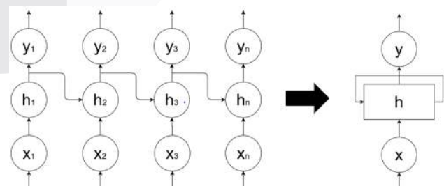
GAMBAR 2.3 ARSITEKTUR SEDERHANA RNN
