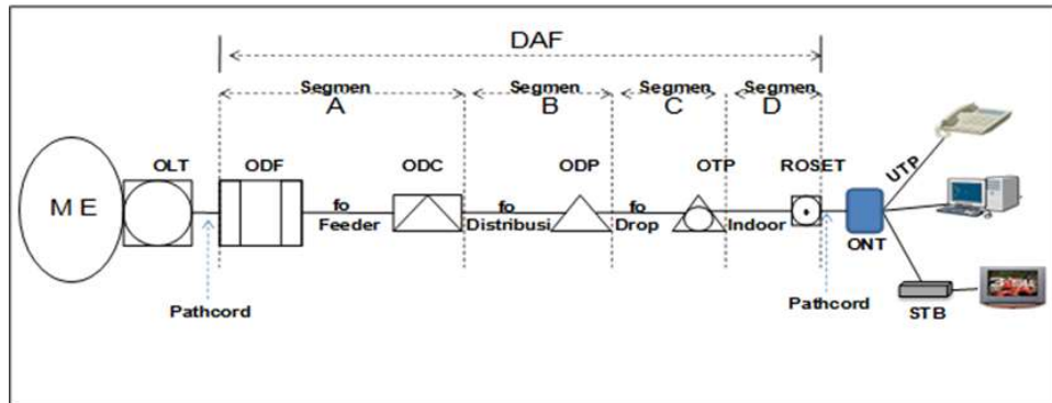
Gambar 1.1 Arsitektur jaringan komunikasi PON
