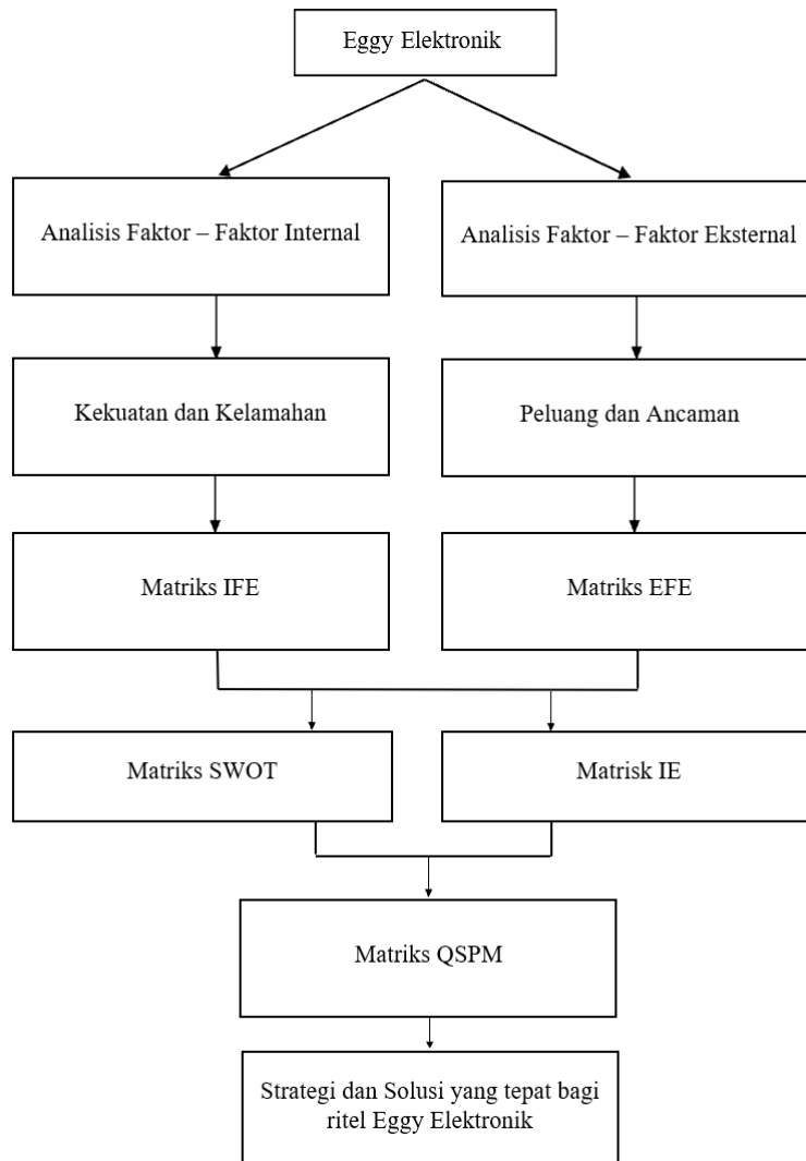
Gambar 2. 1 Kerangka Pemikiran
