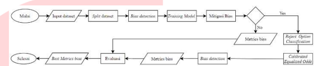
GAMBAR 4 Flowchart post-processing pada mitigasi bias
