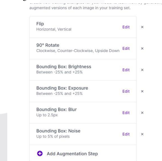
GAMBAR IV.5. Augmentasi Dataset
