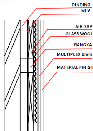
Gambar 7 Pemasangan panel akustik Sumber: Ilustrasi pribadi, 2023
