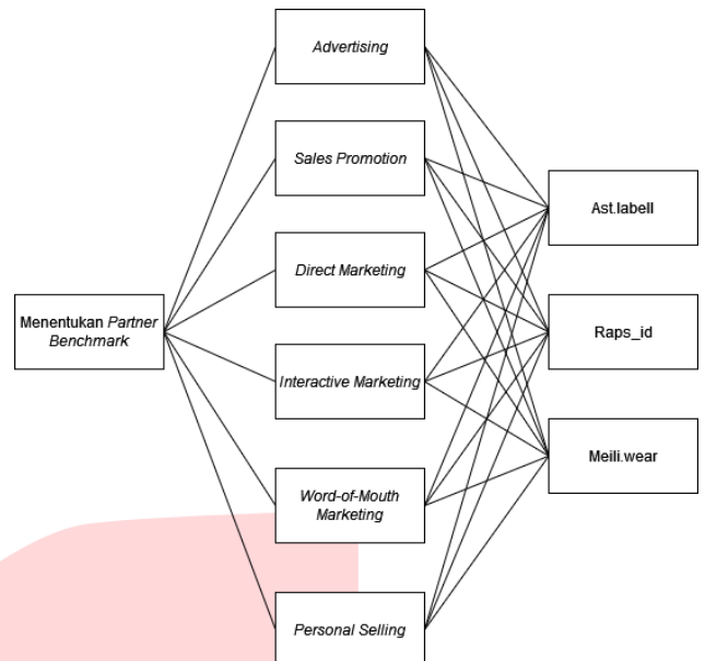
GAMBAR 4 Struktur AHP
