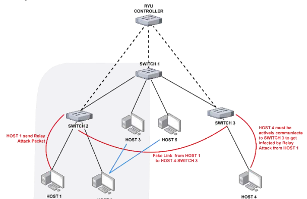
GAMBAR 1, TOPOLOGI JARINGAN(A)
