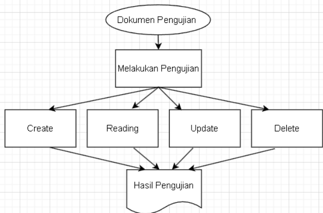
Gambar 3.1 Flowchart Pengerjaan
