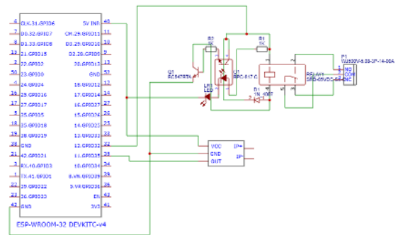
GAMBAR 6 Skematik Rangkaian
