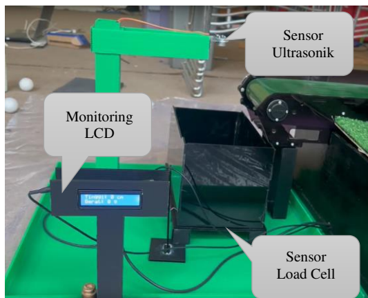
GAMBAR 5 Hasil Integrasi Akhir Sistem
