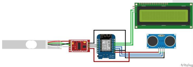
GAMBAR 2 Skema Rangkaian
