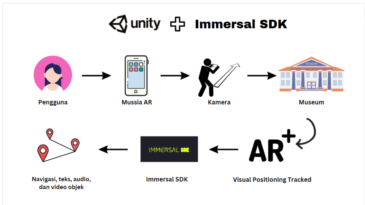
Gambar 3. 1 Arsitektur Aplikasi
