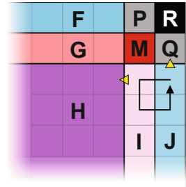
Fig. 7. Livelock pattern
