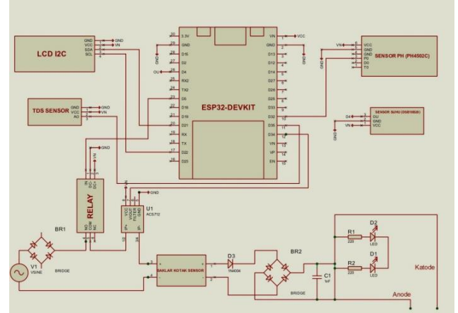
GAMBAR 3.4 Rangkaian Listrik Sistem
