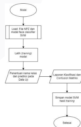
GAMBAR 2 (Flowchart pelatihan)
