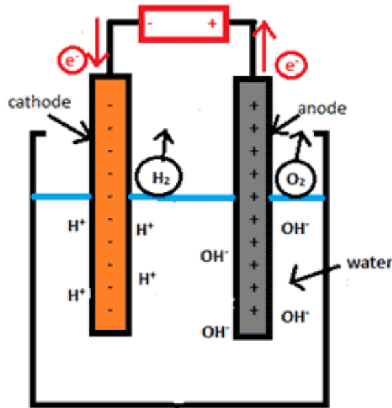
Gambar 1.1 Proses Elektrolisis
