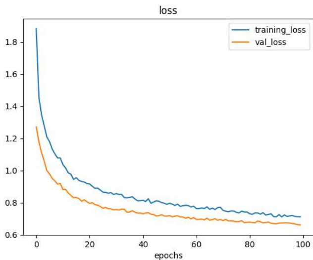
GAMBAR 4.1: Nilai Loss dari Model
