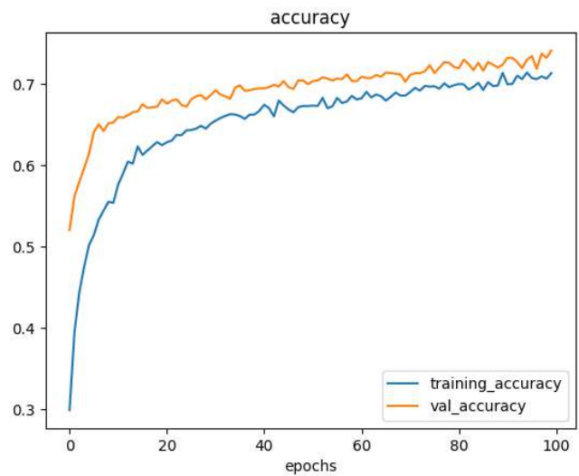
GAMBAR 4.2: Grafik Akurasi dataset
