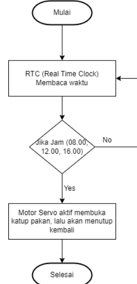
GAMBAR 3 (E) Sistem Kerja Motor Servo
