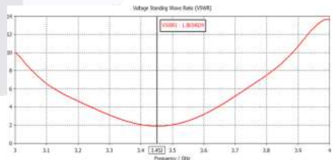
Gambar 3. 3 Hasil simulasi nilai VSWR
