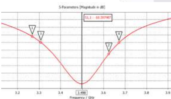
Gambar 3. 6 Hasil simulasi nilai Return Loss optimasi
