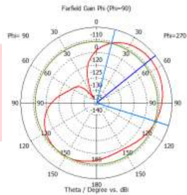
Gambar 3. 8 Sudut Azimuth ( \Phi ) Optimasi
