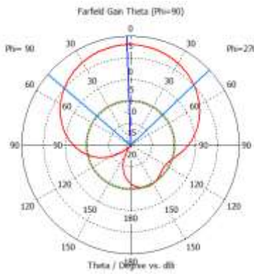
Gambar 3. 5 Sudut Elevasi ( \Theta )
