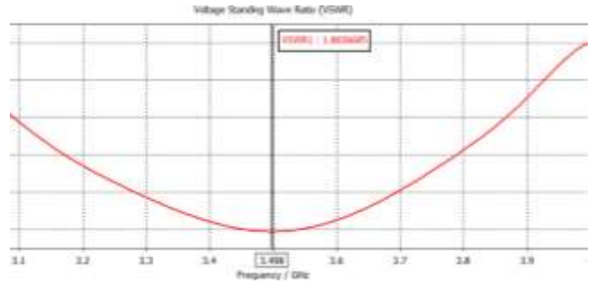
Gambar 3. 7 Hasil simulasi nilai VSWR optimasi
