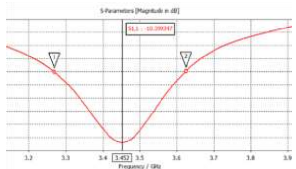
Gambar 3. 2 Hasil simulasi nilai Return Loss
