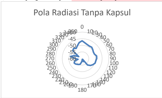
Gambar 26 Hasil Pengukuran Pola Radiasi tanpa Kapsul
