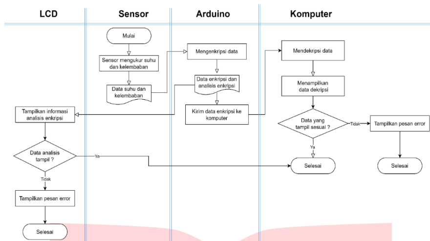
GAMBAR 6. Alur Implementasi Enkripsi
