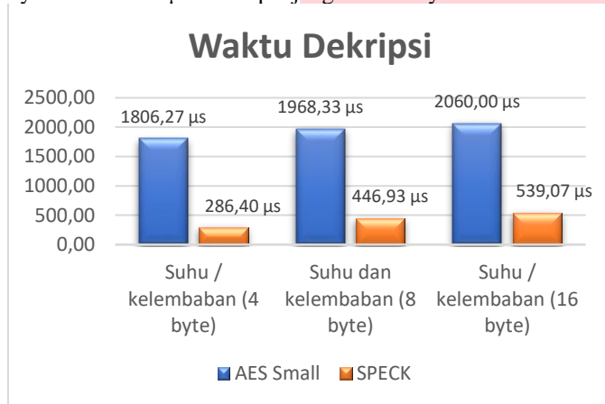
GAMBAR 9. Statistik Waktu Dekripsi
