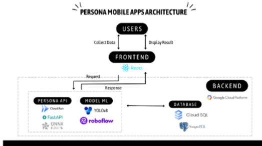
Gambar 1 Arsitektur aplikasi identifikasi kepribadian
