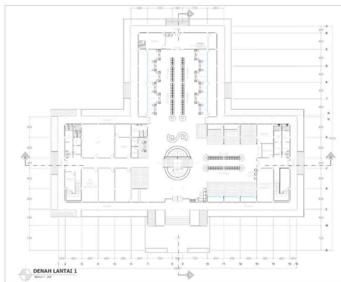
Gambar 1.2 Denah Mal Pelayanan Publik Kota Payakumbuh (sumber : denah arsitek)
