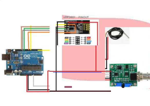
GAMBAR 3.1 Rangkaian Transmitter pada sensor
