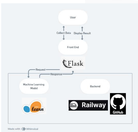
Gambar 1 Rancangan Sistem
