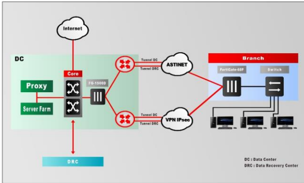
GAMBAR 8. Topologi Jaringan.
