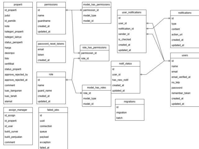
Gambar 2. Struktur Data SQLite
