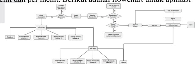
GAMBAR 2. Flowchart Aplikasi
