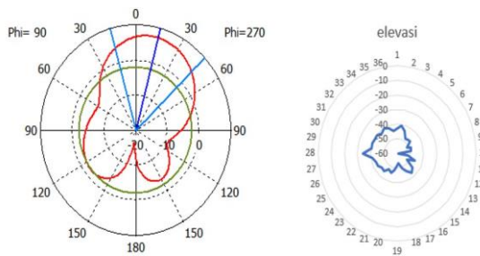
GAMBAR 3 Polarisasi elevasi antenna dengan metasurface
