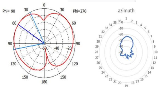
GAMBAR 4 Polarisasi azimuth antenna dengan metasurface
