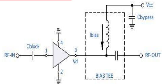
GAMBAR 1 Skematik LNA
